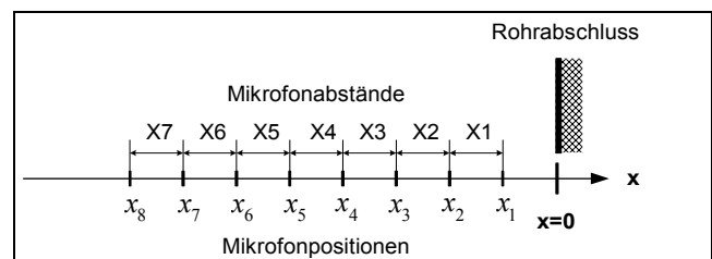
Abbildung 2: Mikrofonpositionen und -abstände in Bezug auf den Rohrabchluss
