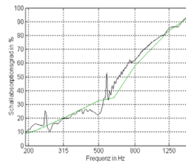
Abbildung 6: Gemessener Schallabsorptionsgrad der Schaumstoffprobe (schwarz) verglichen mit den Angaben des Herstellers (grün).
