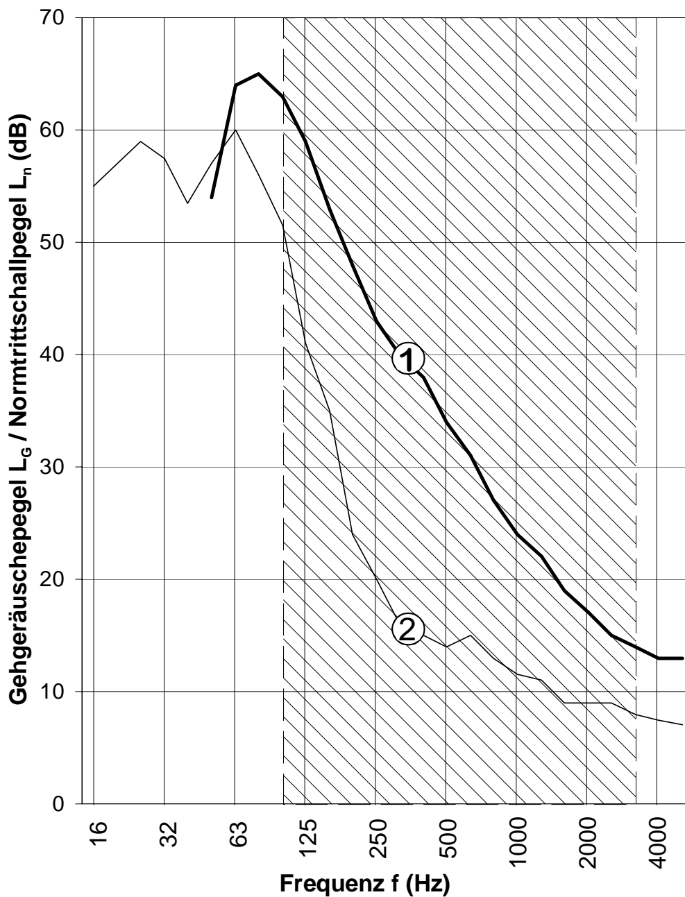
Diagramm 1: Gehgeräusche-Immissionen und Trittschalldämmung bzw. Normtrittschallpegel einer mehrschaligen Geschossdeckenkonstruktion aus Holz
