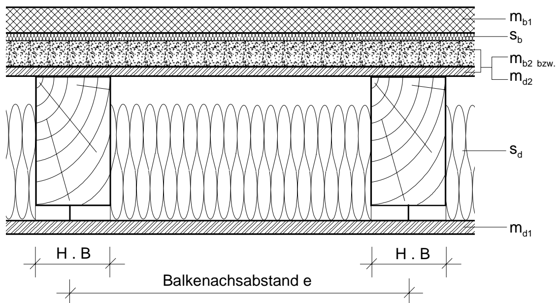
Schnitt durch Geschossdecke mit eingetragenen Grössen
