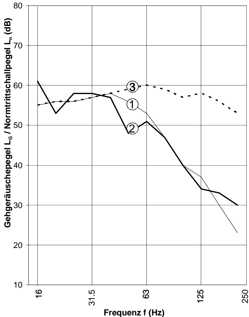
Diagramm 2: Darstellung des Gehgeräuschepegels L_G und des Normtrittschallpegels L_n
