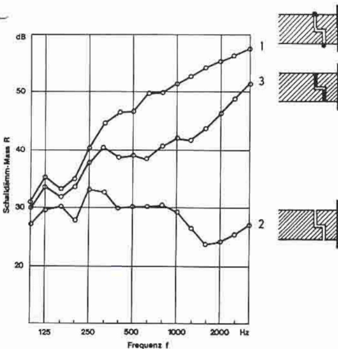
Diagramm 1: Darstellung der Luftschalldämmung R einer Türanordnung mit verschiedenen Fugenausbildungen. Kurve 1: Türblatt allein; Kurve 2: Türe mit offener Fugenausbildung; Kurve 3: mit bedämpfter Fugenausbildung (Filzstreifen).
