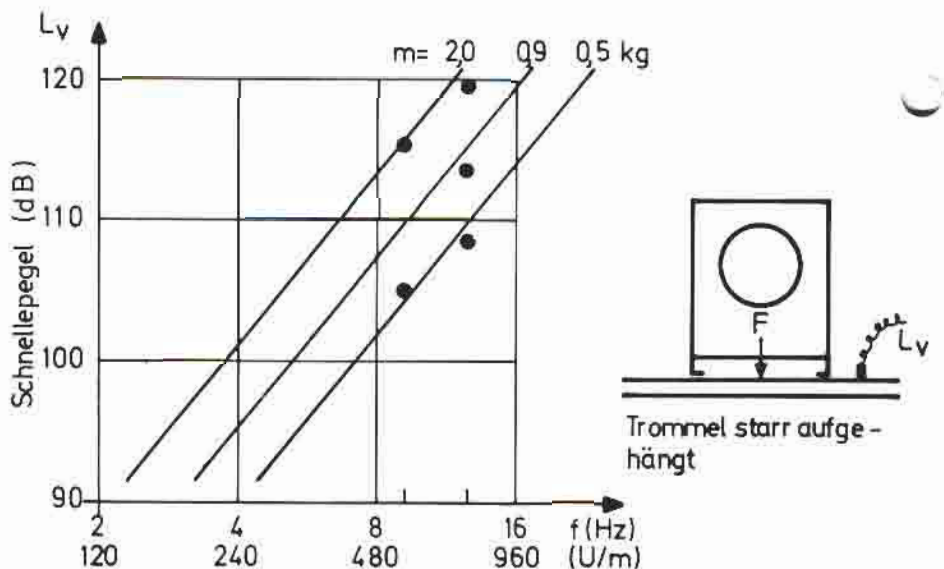
Diagramm 1: Darstellung der auf einer 160 mm dicken Stahlbetondecke ( S = 18 m 2 ) ermittelten Schwingungspegel in Funktion der Wäschetrommel-Tourenzahl; Parameter: Massenumwucht m .
